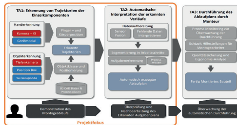
Links: Symbolischer Arbeitsplatz in AI Teach | Oben: Die Inhalte in AI Teach, von Objekterkennung über automatische Interpretation des Erkannten bis zum fertigen Ablaufplan der Montage, Bilder: BIBA GmbH
